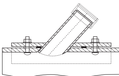
Bild 7-9-2 Sattelstücke 45° - geschraubt
