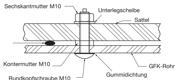
Bild 7-12-3 Detailansicht der Schraubverbindung
