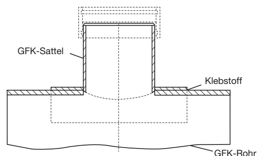
Bild 7-12-6 Sattelstück 90° - geklebt -
