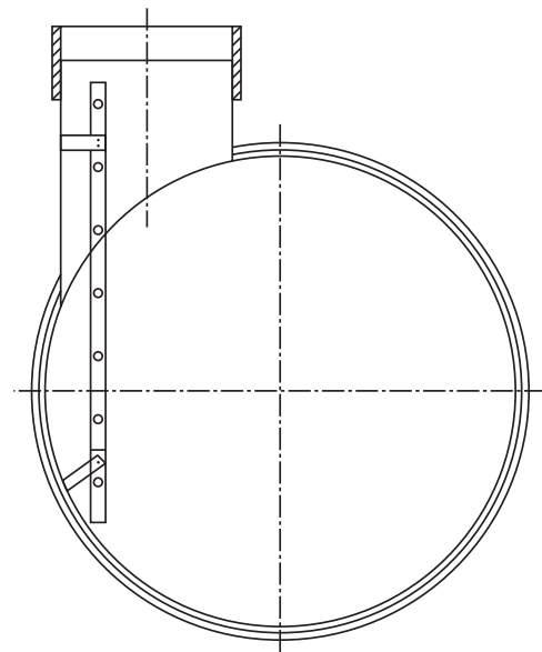
Bild 7-25-2 Tangential-Schacht
