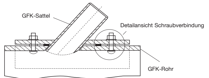
Bild 7-12-1 Sattelstück 45° - geschraubt -
