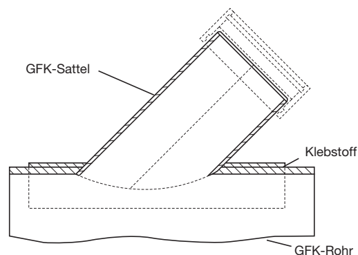
Bild 7-12-5 Sattelstück 45° - geklebt -
