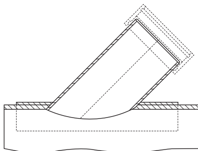
Bild 7-9-4 Sattelstücke 45° - geklebt
