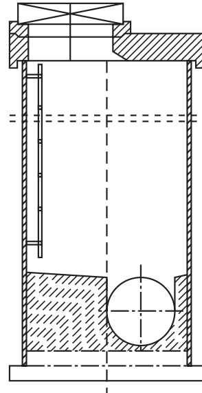
Bild 7-25-1 Standard-Schacht
