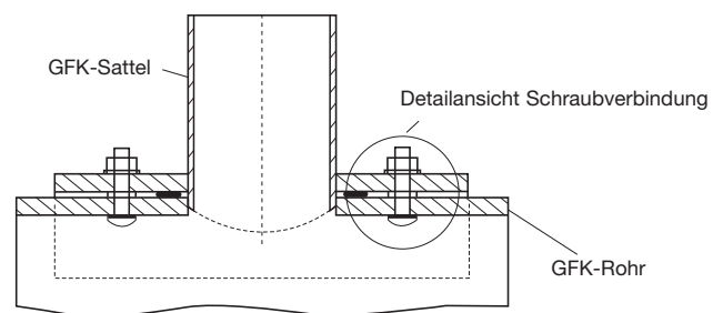
Bild 7-12-2 Sattelstück 45° - geschraubt -
