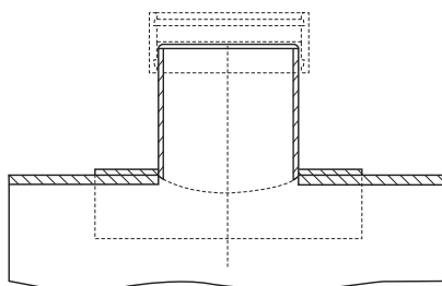
Bild 7-9-3 Sattelstücke 90° - geklebt
