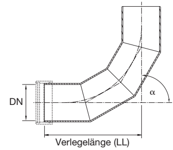
Viersegment-Bogen
