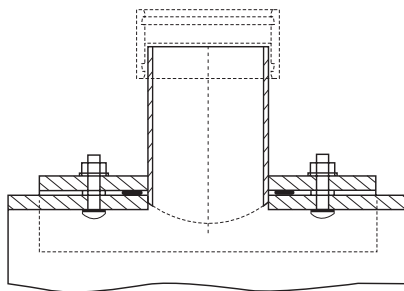
Bild 7-9-1 Sattelstücke 90° - geschraubt
