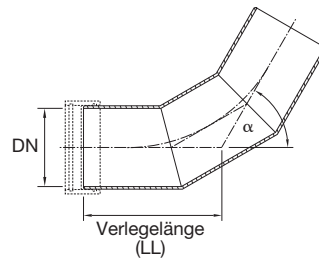
Dreisegment-Bogen
