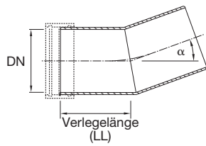
Zweisegment-Bogen
