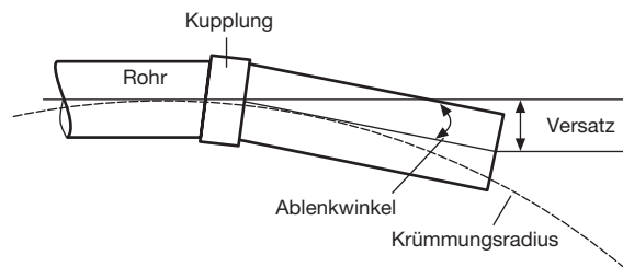
Abbildung 6-1 Versatz und Radius eines Bogens, Kupplung, Rohr, Abwinklung, Versatz, Krümmungsradius
