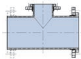
T-Stück 90°
